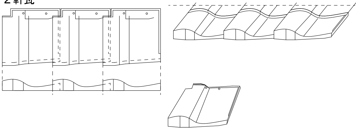
2 軒瓦
