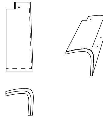
4 右袖瓦
