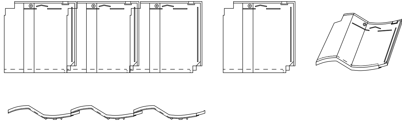
1 棧瓦
