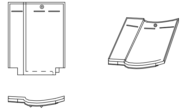
7 半瓦
