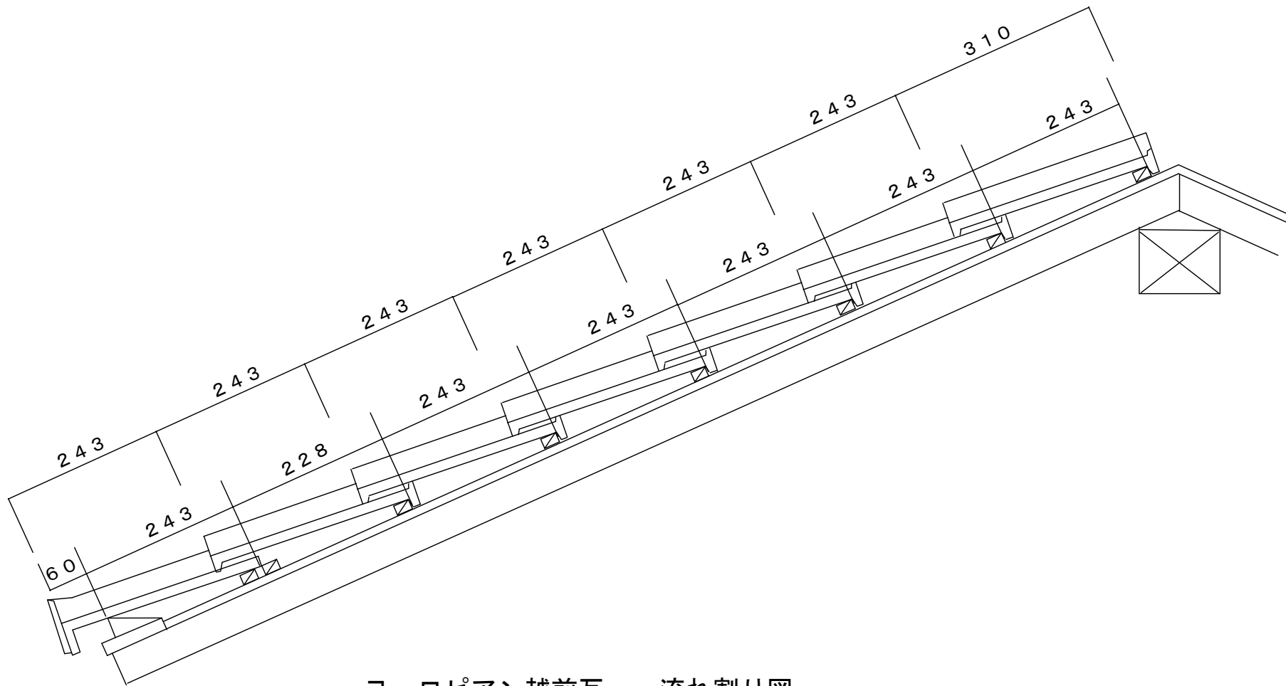
ヨーロッパ越前瓦 流れ割り図
